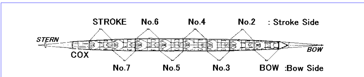
エイトのシートポジション。艇首(バウ)から順番に番号が割り当てられる。
